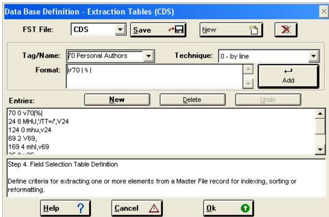
Figure 16 - FST Editor
