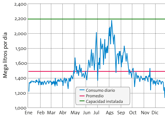
Figura 3. Consumo Diario de Agua en 2001 (ML/d) - (Toronto, 2002)
