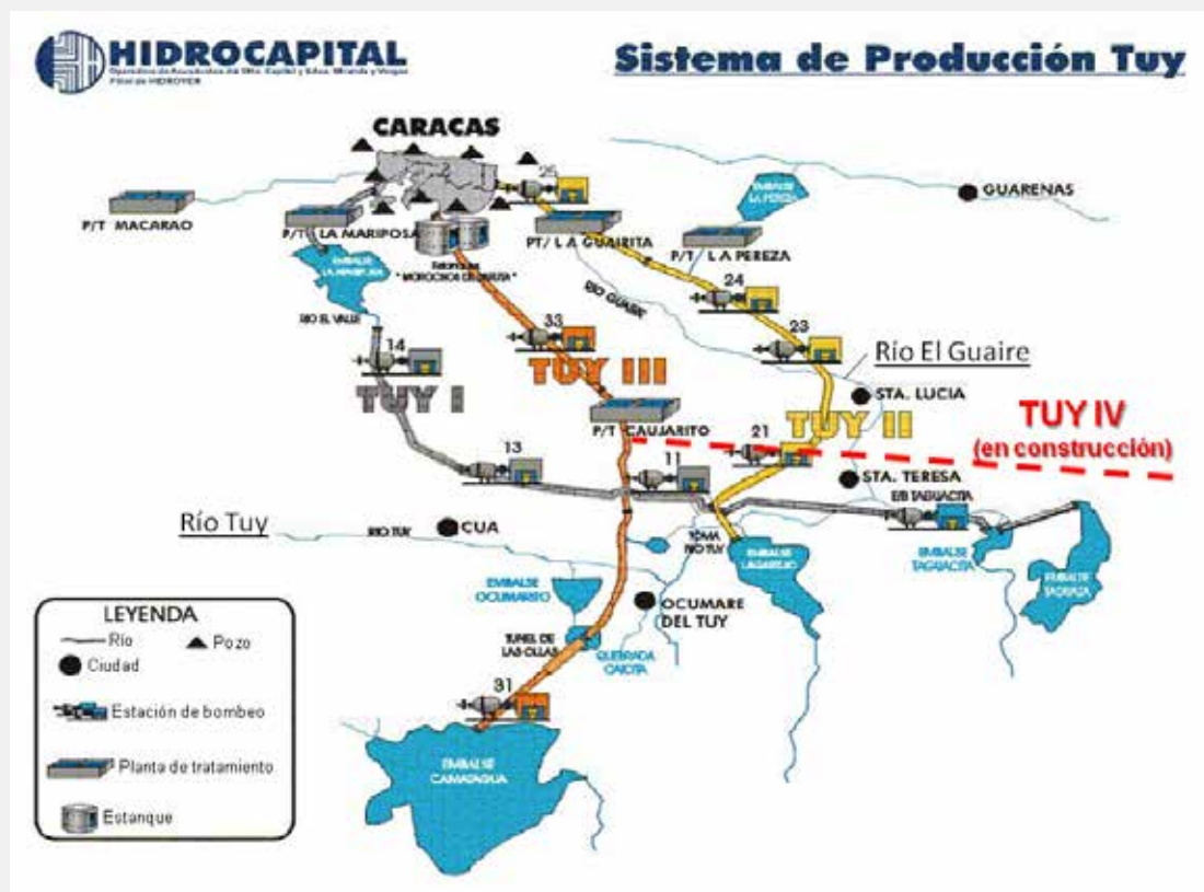
Figura 4. Sistema Tuy. Modificado de HIDROCAPITAL
