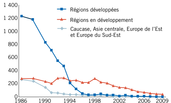
Consommation de substances appauvrissant la couche d'ozone (ODS), 1986-2009 (milliers de tonnes métriques ayant le potentiel de détruire la couche d'ozone)
