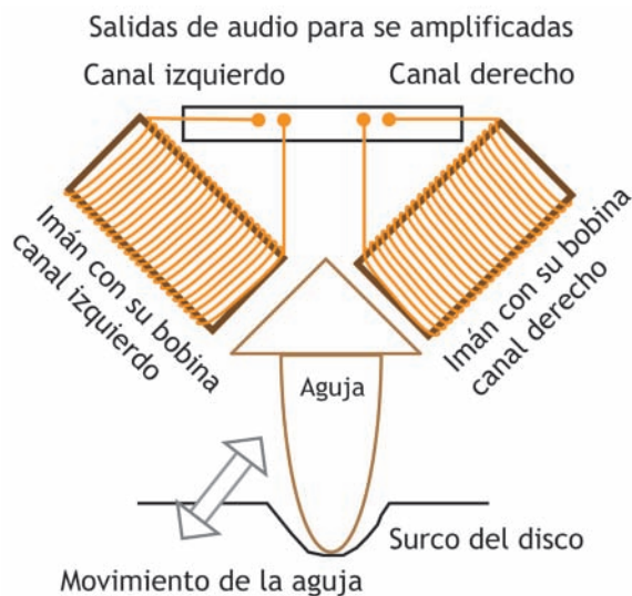
[136] Funcionamiento del tocadiscos estéreo
