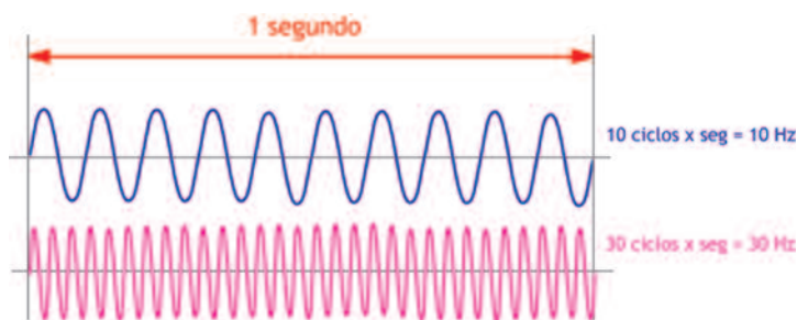
[15] A mayor frecuencia (30 Hz), gráficamente los ciclos se ven más juntos, lo que evidencia la menor longitud de onda.
