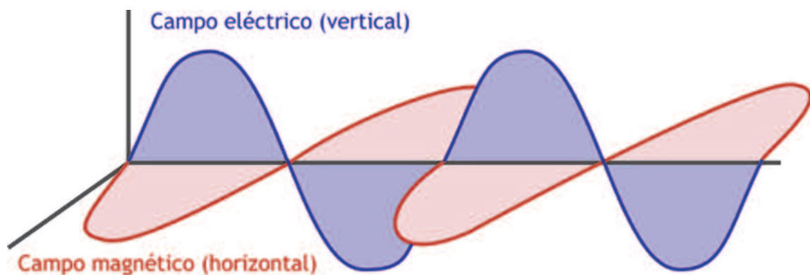
[32] Onda electromagnética
