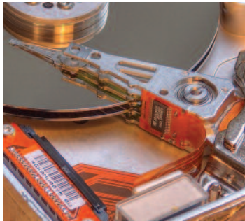
[197] Detalle interno de un HD
