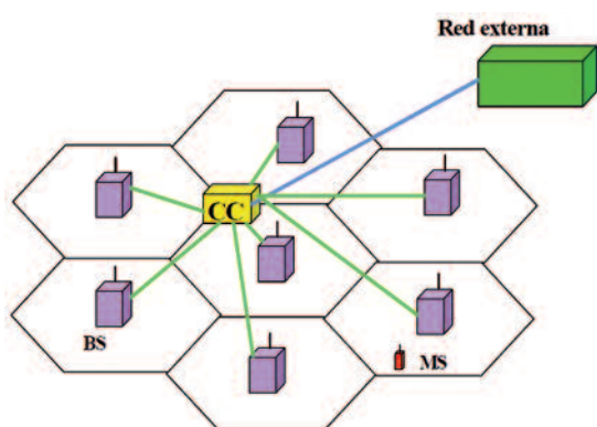
[177] Forma de las celdas cada una con su antena.
