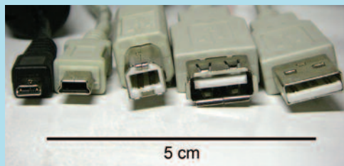
[198] Distintos tipos de conectores USB
