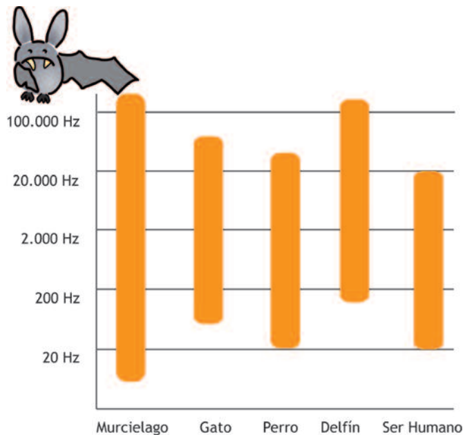
[9] Tabla comparativa de las frecuencias que escuchan los animales y el ser humano.
