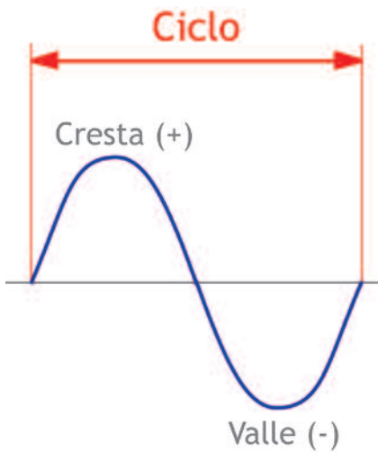
[5] Representación de un ciclo completo de onda.
